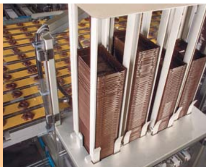
Trays werden einem Hochleistungsmagazin entnommen und zugeführt
